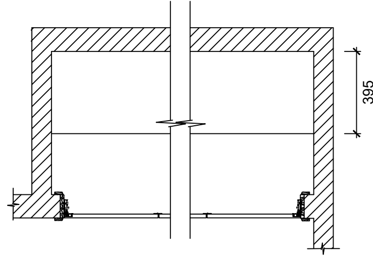
OPK Bi-fold Door Architrave Door Jamb Top View
